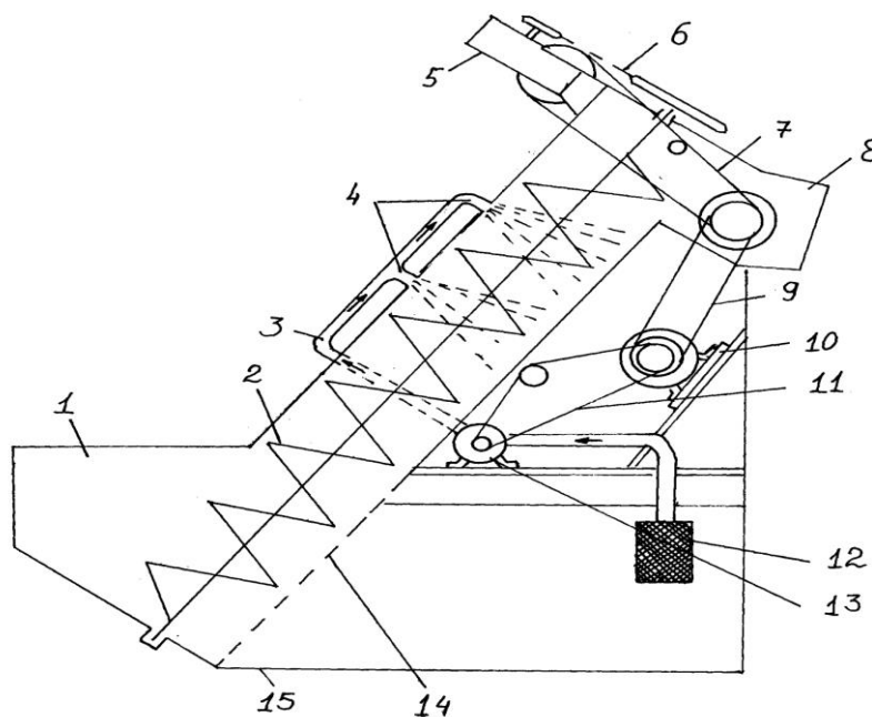
Рисунок 2.1.2 - Технологическая схема измельчителя ИКС-5М:
