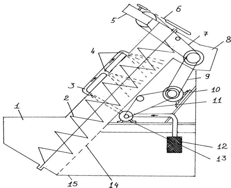
Рисунок 2.1 - Технологическая схема измельчителя ИКС-5М:
